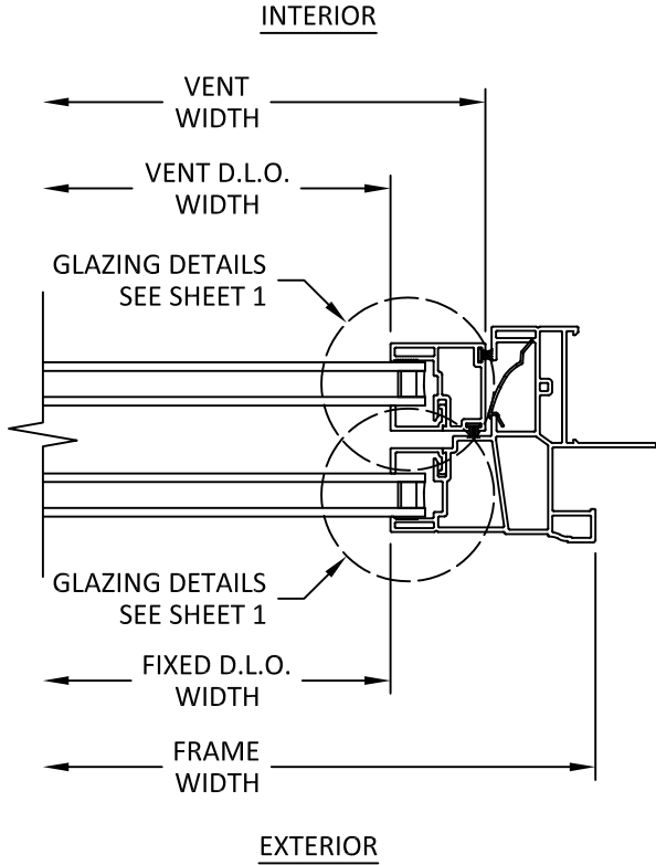
E 4 HORIZONTAL SECTION JAMB
